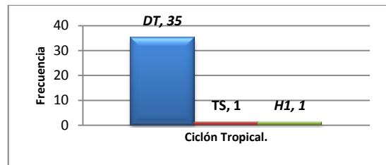
Figura 4: Ciclones tropicales en radio de 500 km de las costas salvadoreñas
