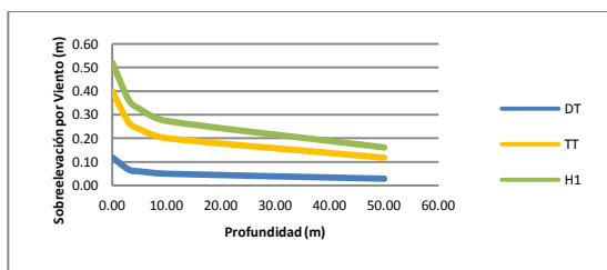
Figura 7: Sobrelevación por viento para distintas profundidades
